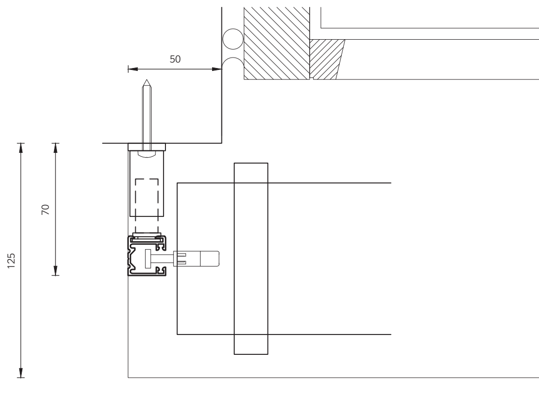
Vandret snit 1:2
