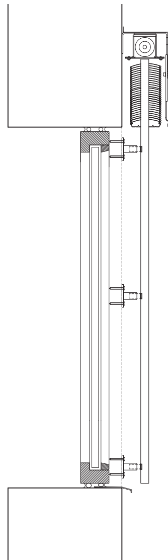
Lodret snit 1:10
