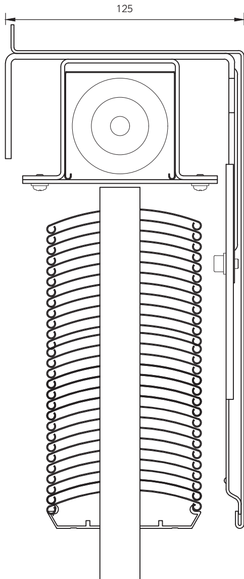
Lodret snit 1:2
